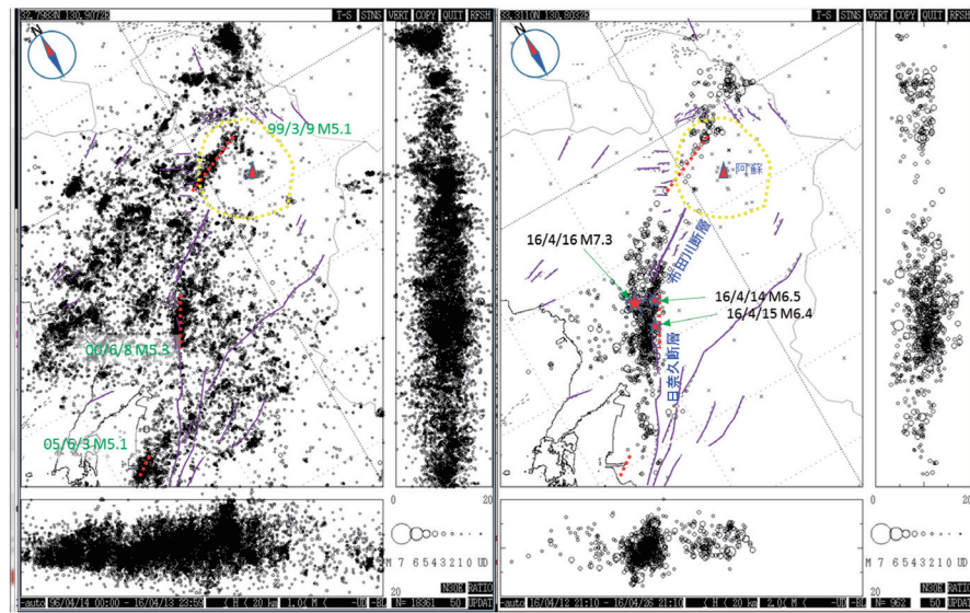
2016年4月14日M6.5前20年間の活動と発生後4月26日までの地震活動。震源分布の平面図と鉛直断面図を示す。図中の△、赤線、紫線は火山、20年以内のM5以上の震源、活断層を示す。黄色線は阿蘇カルデラのおおむねの位置。発生前、後の震源は九州大学、2016年熊本地震合同地震観測グループによる。
